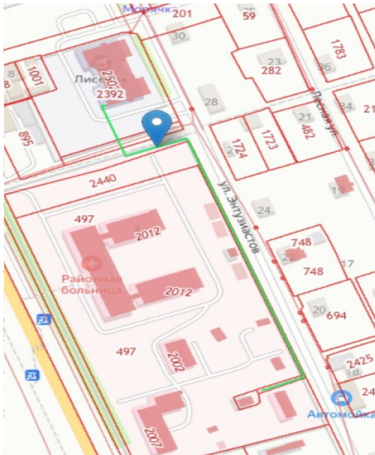
Схема тепловой сети к детскому саду «Лисенок»
